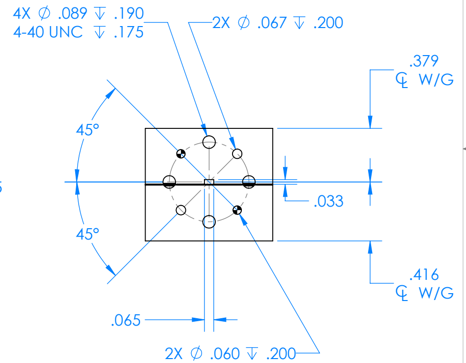
UG-387 FLANGE
