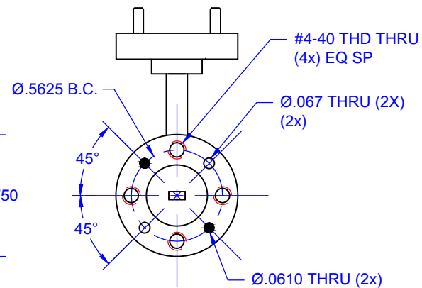
UG-387 FLANGE
