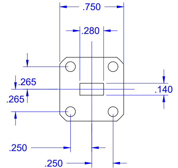
UG 599 FLANGE
