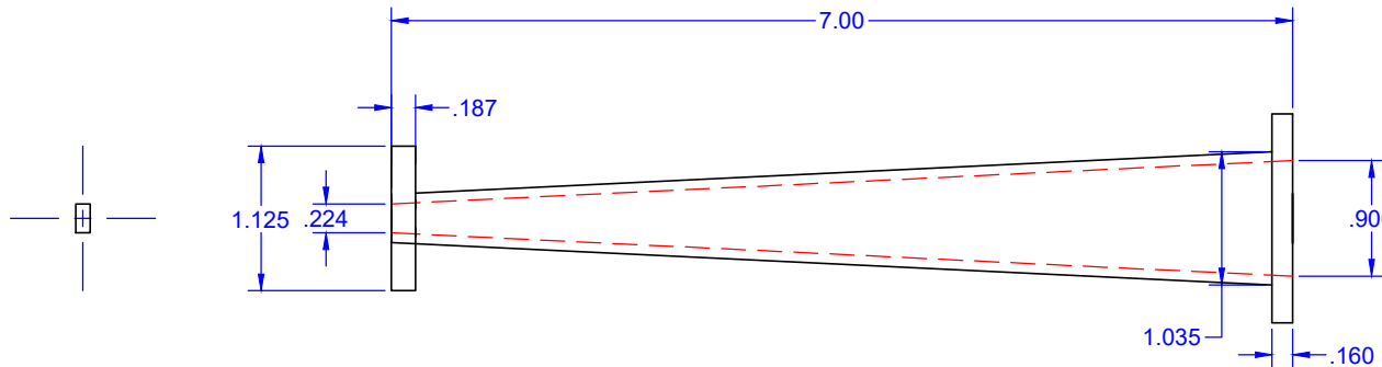
UG-383 FLANGE
