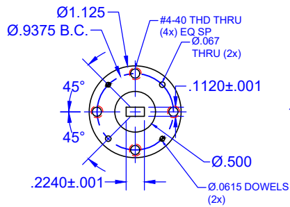
UG-383 FLANGE
